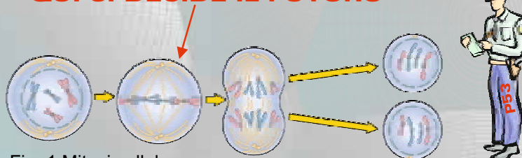
Fig. 1 Mitosi cellulare
